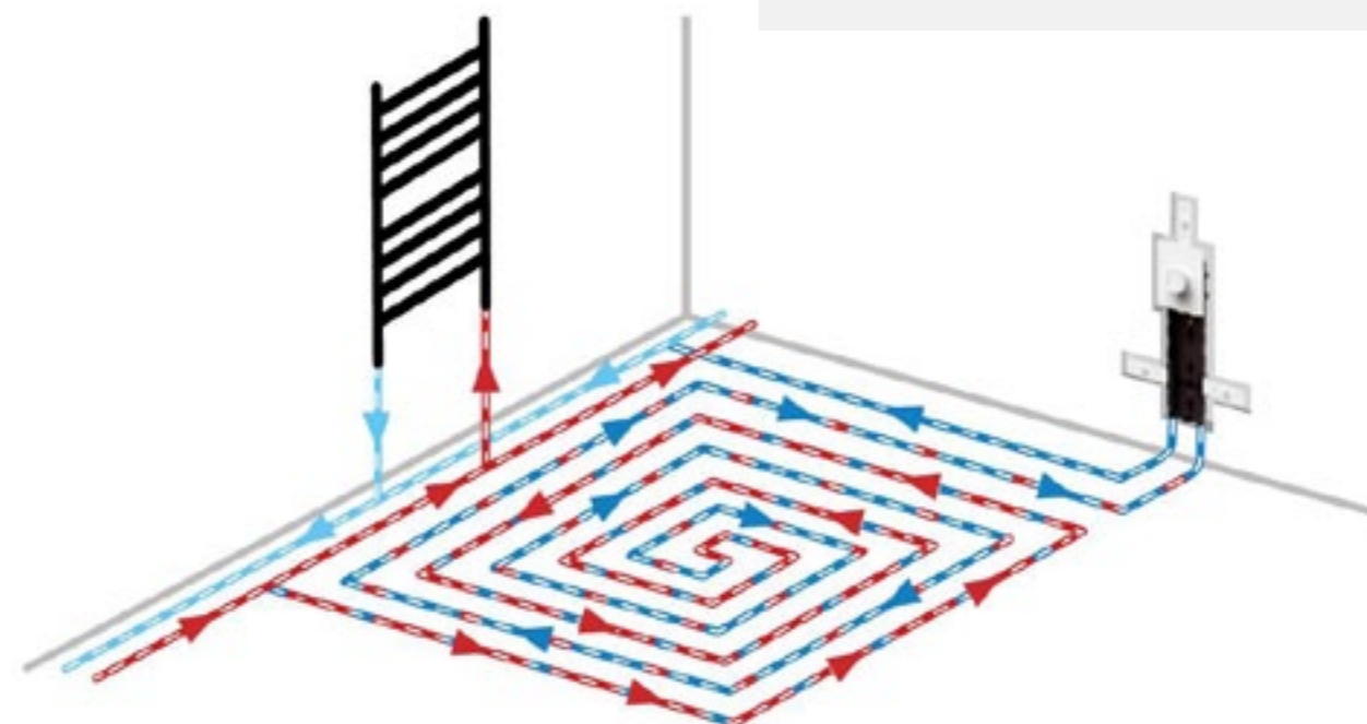
Przykładowy schemat aplikacyjny zestawu RTL-Box 324 Vario
