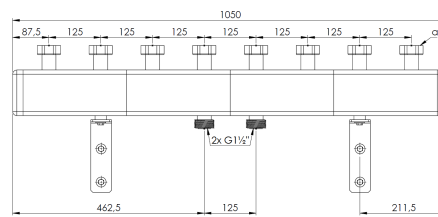
(a) - 8x nakrętka G1½"
