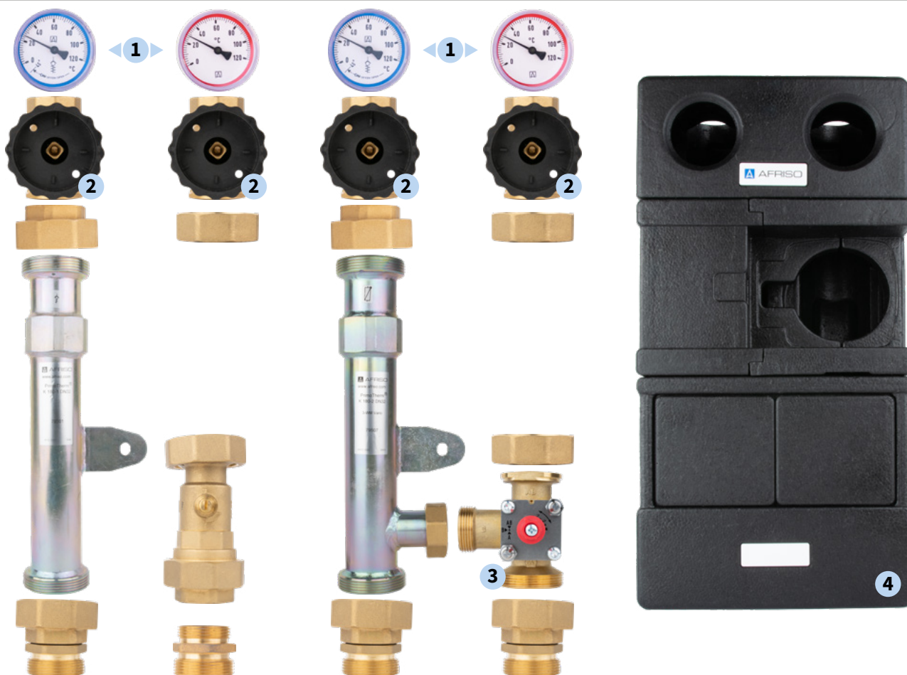
PrimoTherm K 180-2 DN32, zawór mieszający, siłownik 343, bez pompy
