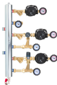
BPS na 3 obiegi z pompami Grundfos UPM3
