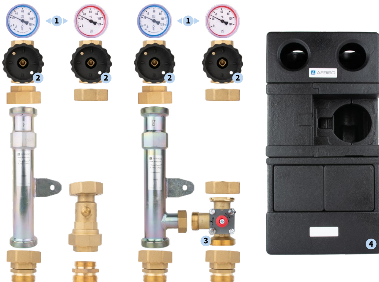
PrimoTherm K 180-2 DN32, zawór mieszający, siłownik ARM 343, bez pompy
