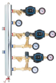
BPS na 3 obiegi z pompami AFRISO APH
