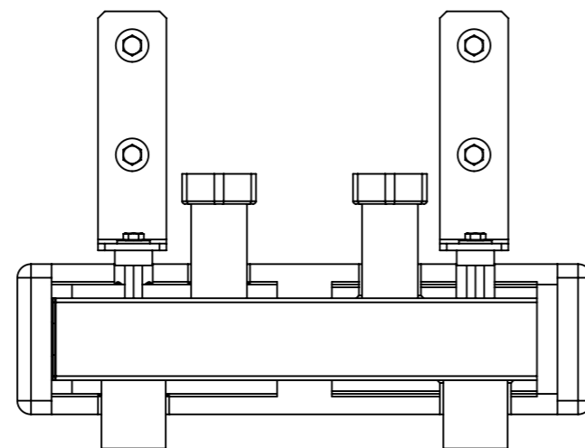
Sprzęgło hydrauliczne do rozdzielacza KSV bez przedniej części izolacji
