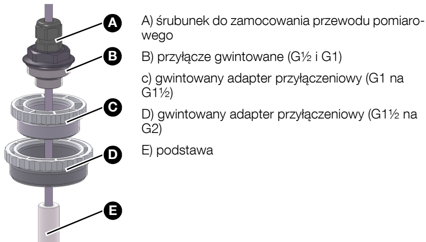
Abbildung 9: Zestaw śrubunków do przewodu
