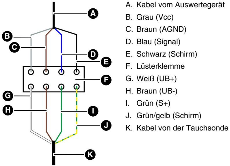
Abbildung 7: Anschluss Lüsterklemme
