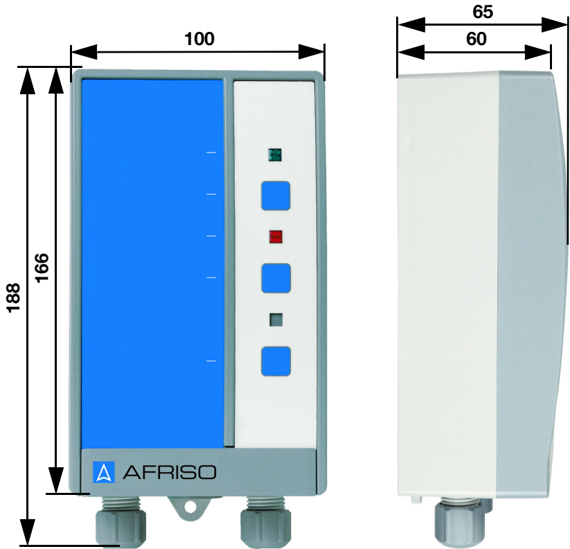
Abbildung 2: Wymiary w mm
