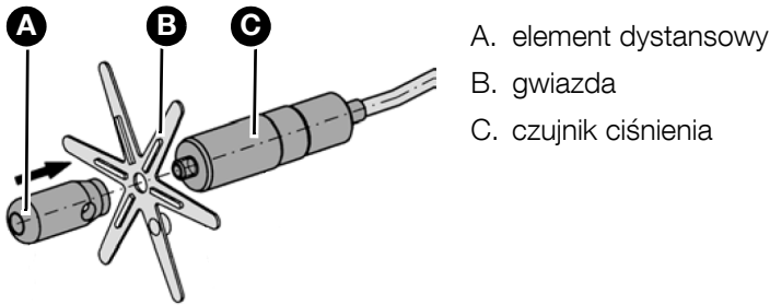
Abbildung 8: Montaż sondy zanurzeniowej
