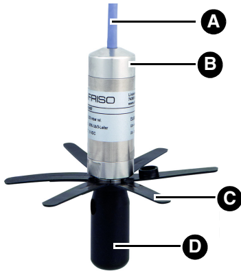
Abbildung 3: Tauchsonde
