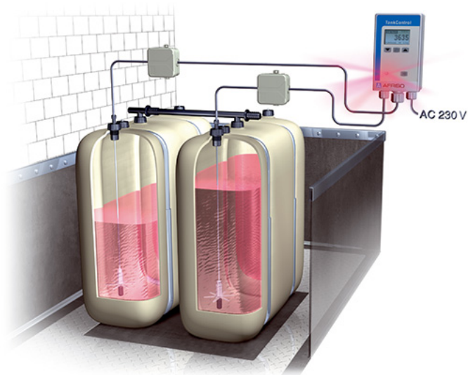
Abbildung 6: Pomiar poziomu napelnienia z rejestracją różnicy w baterii zbiorników
