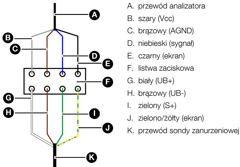
Abbildung 7: Podłączenie listwy zaciskowej
