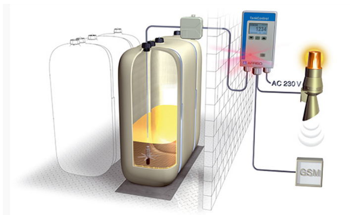
Figure 5: Mesure de niveau de remplissage avec une sonde à immersion
