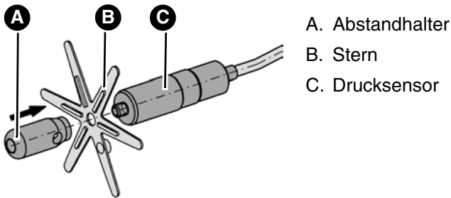
Abbildung 8: Tauchsonde montieren
