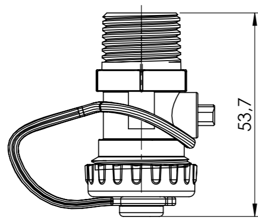
Zawór spustowy
