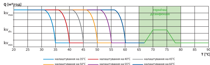
Рис. 11. Графік зміни Kv для клапанів АТВ 200 і АТВ 210
