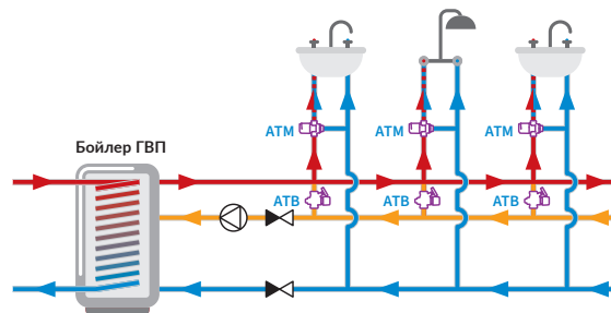
Рис. 6. Клапани АТВ, використовувані в циркуляційній системі у вертикальному виконанні з термостатичними клапанами АТВ
