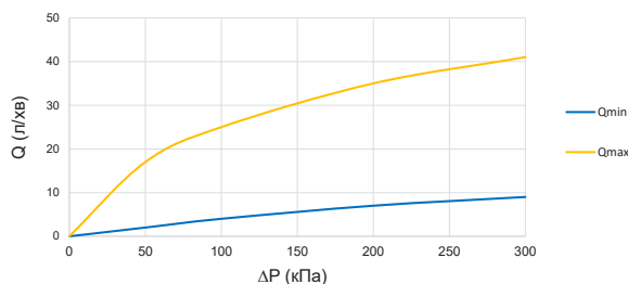
Рис. 12. Характеристика потоку для клапанів АТВ 100 і АТВ 110
