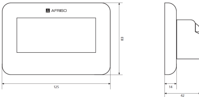
Рисунок 3. Размеры термостата RT05 F
