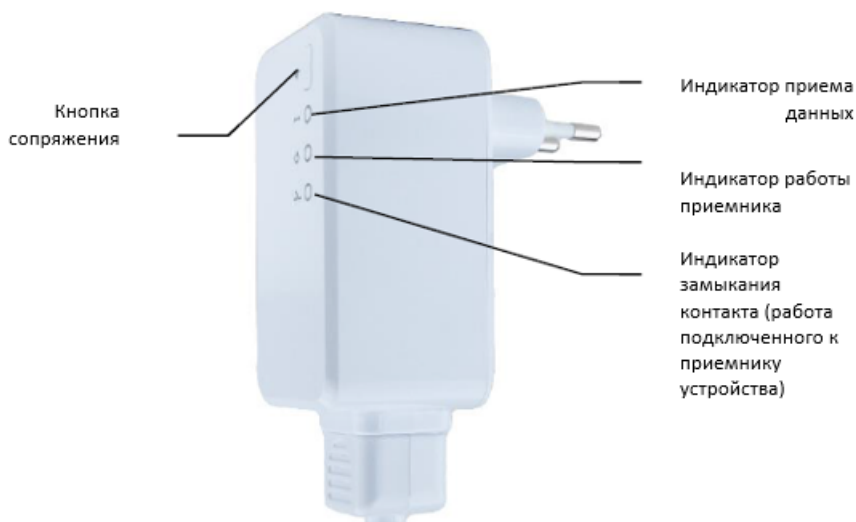
Рисунок 4. Приемник беспроводного сигнала с контактом
