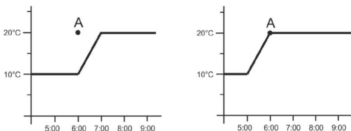
Рисунок 18. Слева график температуры в помещении без использования алгоритма «Оптимальный пуск», справа – с использованием
