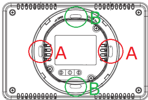
Рисунок 6. Монтажные отверстия
