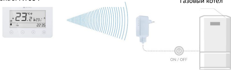
Рисунок 5. Пример схемы применения – Программируемый комнатный термостат RT05 F используется для управления газовым котлом
