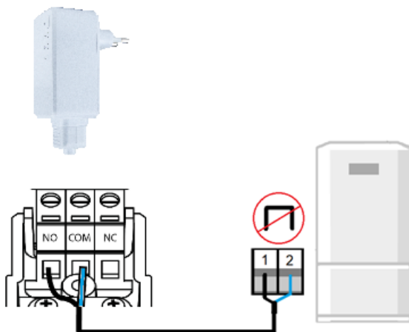
Рисунок 7. Пример электрического подключения приемника термостата RT05 F к газовому котлу
