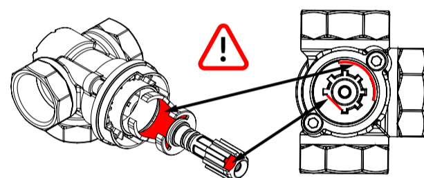
Abb. 2 Position des Verschlusselements in Bezug auf die Abflachung auf dem Adapter und der Ventilspindel
