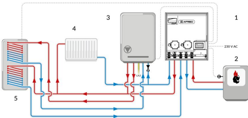
Rysunek 6: Przykładowy schemat aplikacyjny – połączenie kotła gazowego z kominkiem na pellet przy zastosowaniu PrimoBox AHB 620 lub 622
