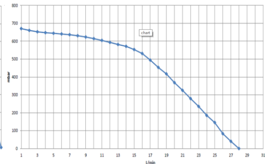
Rysunek 9: Wykresy natężenia przepływu przez bieg pierwotny (z lewej) i bieg grzewczy (z prawej) zestawu separacyjnego AHB 622 z zaworem termostatycznym ATV 213. Oś pionowa: wysokość podnoszenia pompy [mbar]. Oś pozioma: przepływ [l/min]
