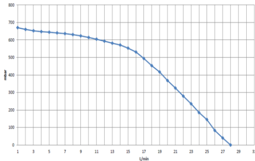
Rysunek 8: Wykresy natężenia przepływu przez bieg pierwotny (z lewej) i bieg grzewczy (z prawej) zestawu separacyjnego AHB 620. Oś pionowa: wysokość podnoszenia pompy [mbar]. Oś pozioma: przepływ [l/min]
