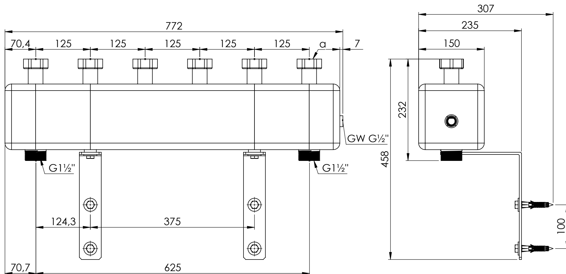
(a) - 6x nakrętka G1½"
