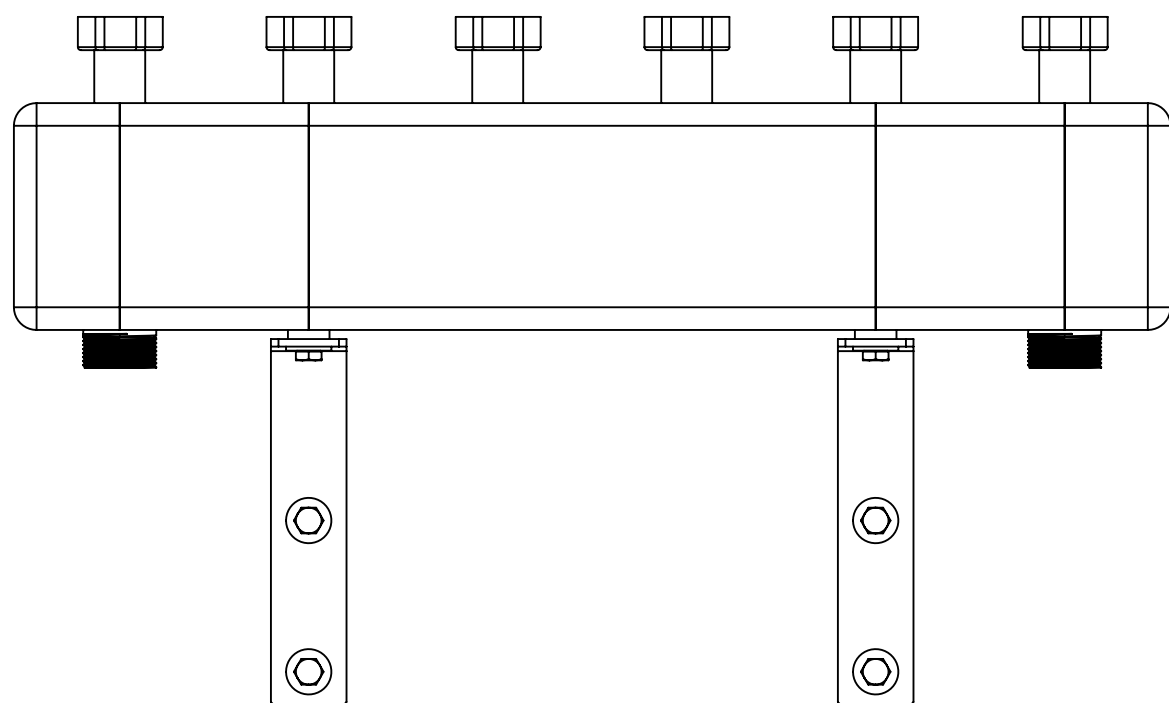
Rozdzielacz ze sprzęgłem hydraulicznym KSV 125-2 bez przedniej części izolacji
