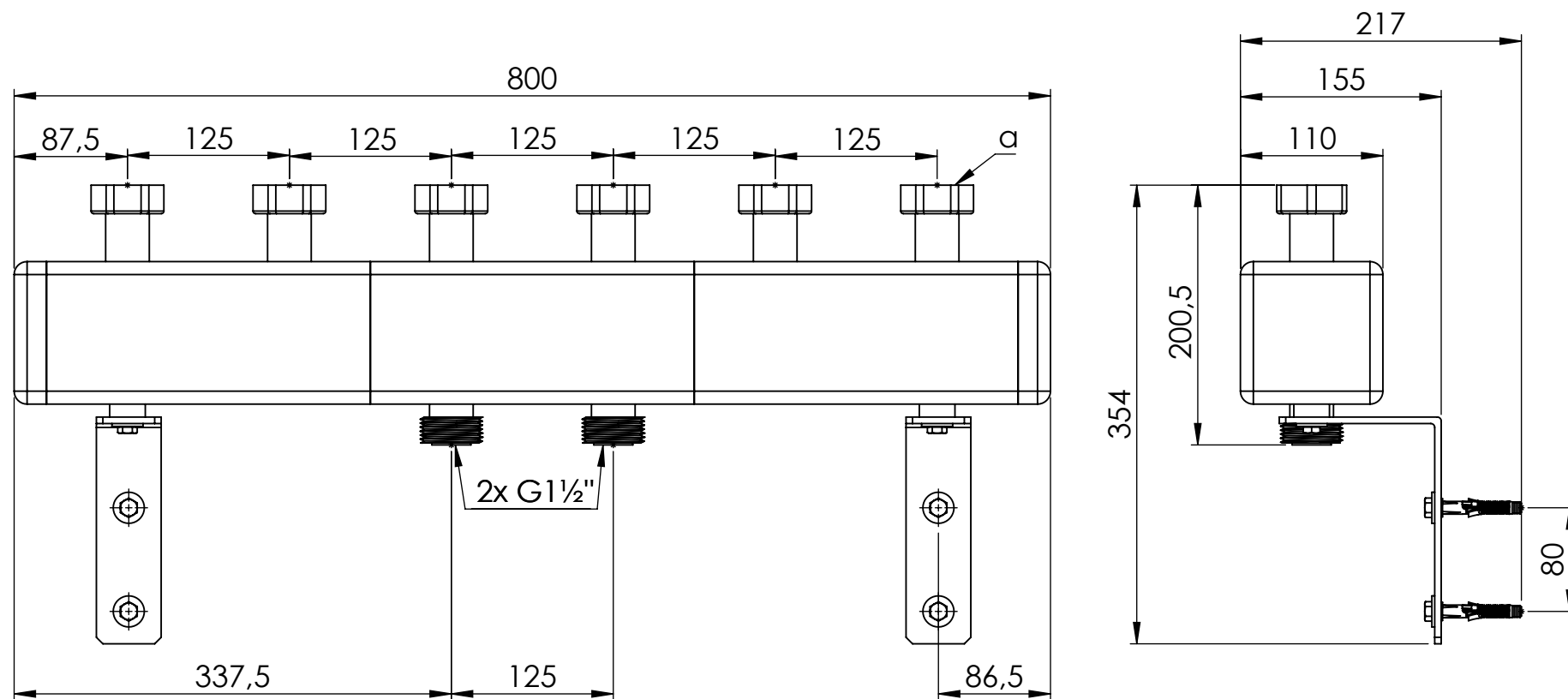
(a) - 6x nakrętka G1 1/2"
