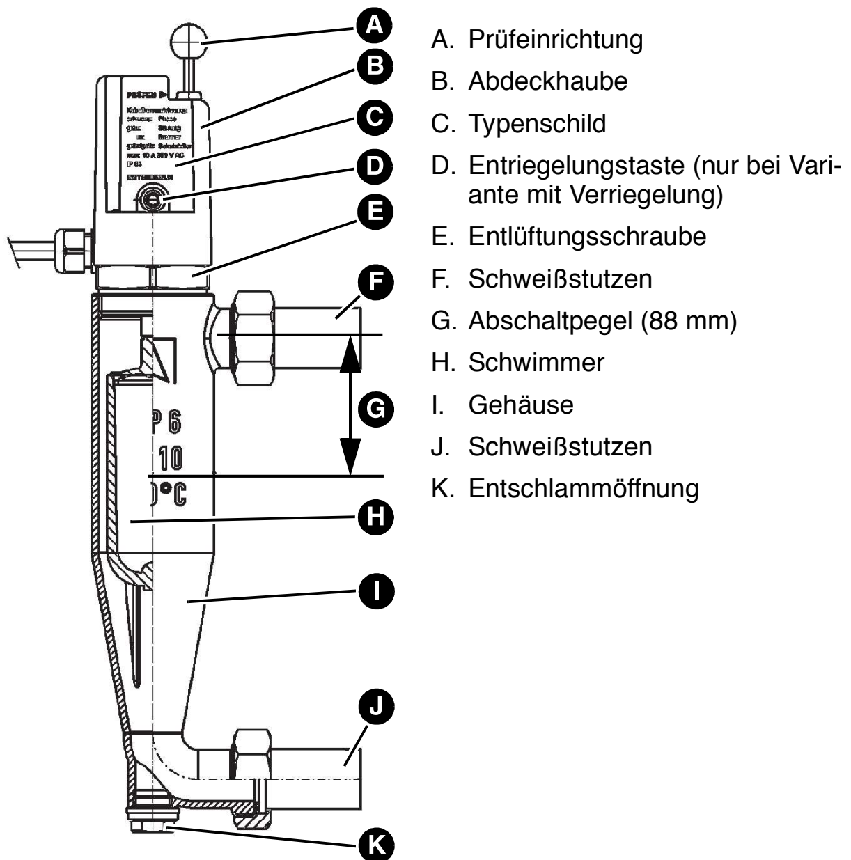
Abbildung 1: Aufbau WMS-WP6
