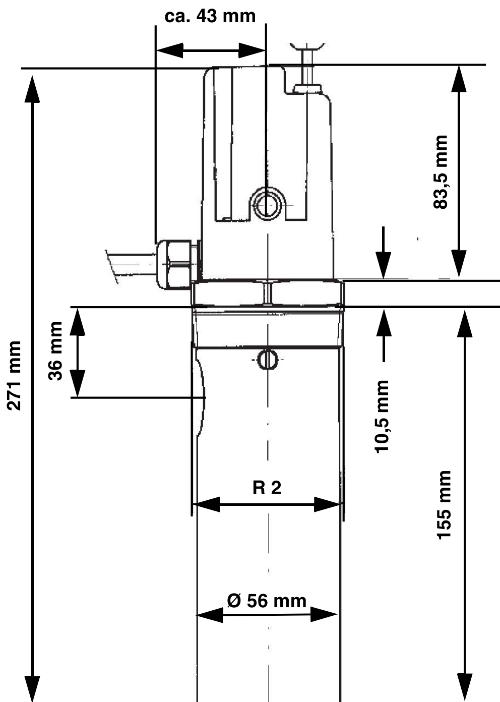
Figura 4: WMS-WP6 con pozzetto corto
