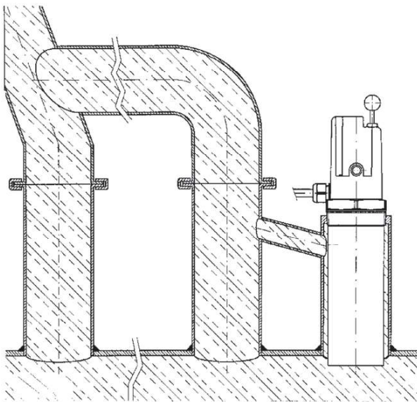
Ilustracja 6: WMS-WP6 z krótką rurą ochronną
