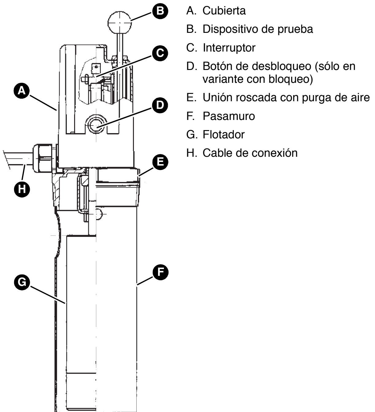
Figura 2: WMS-WP6 con pasamuro corto
