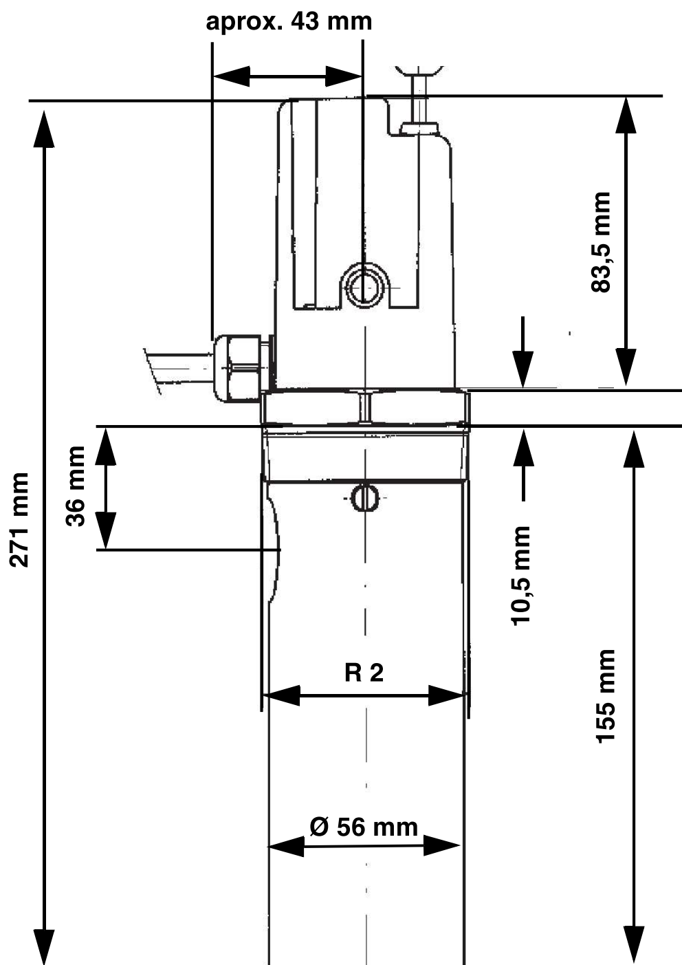
Figura 4: WMS-WP6 con pasamuro corto
