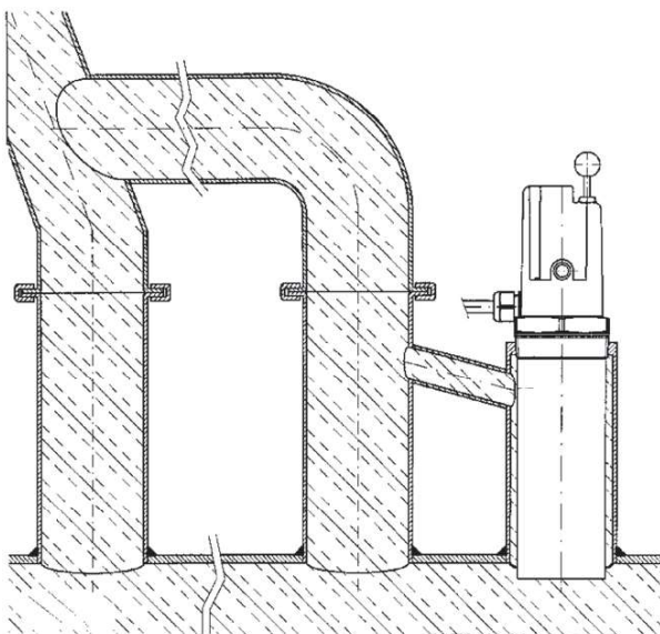
Figure 6: WMS-WP6 avec tube de protection court
