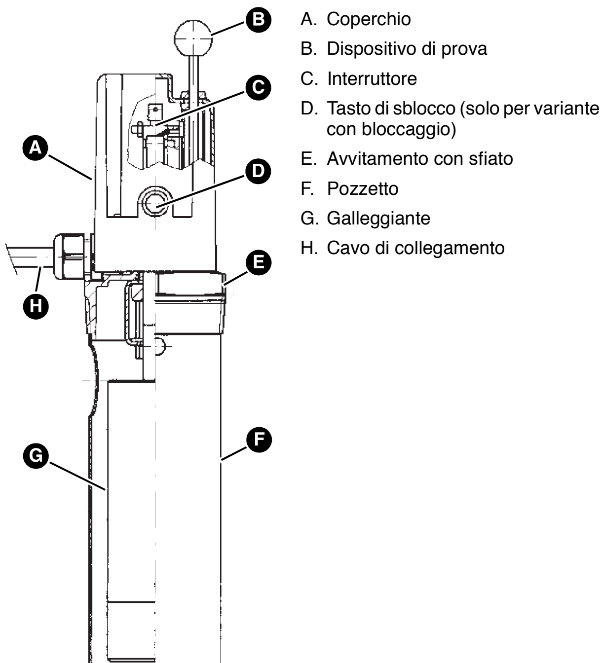
Figura 2: WMS-WP6 con pozzetto corto
