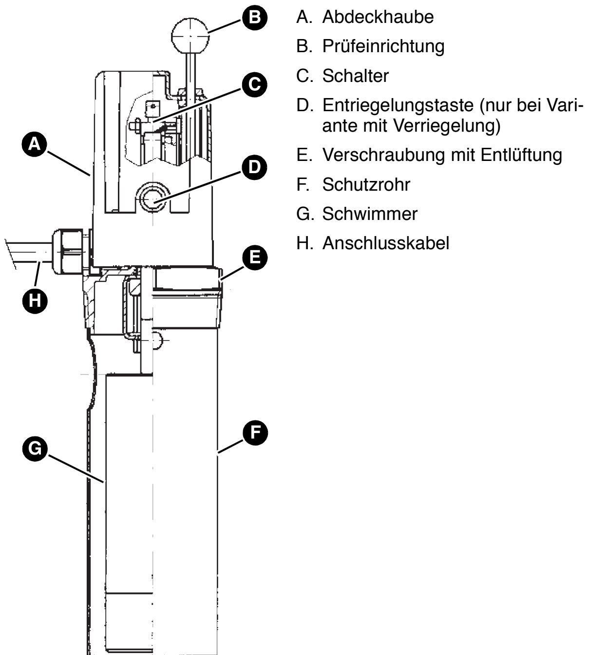
Abbildung 2: WMS-WP6 mit kurzem Schutzrohr
