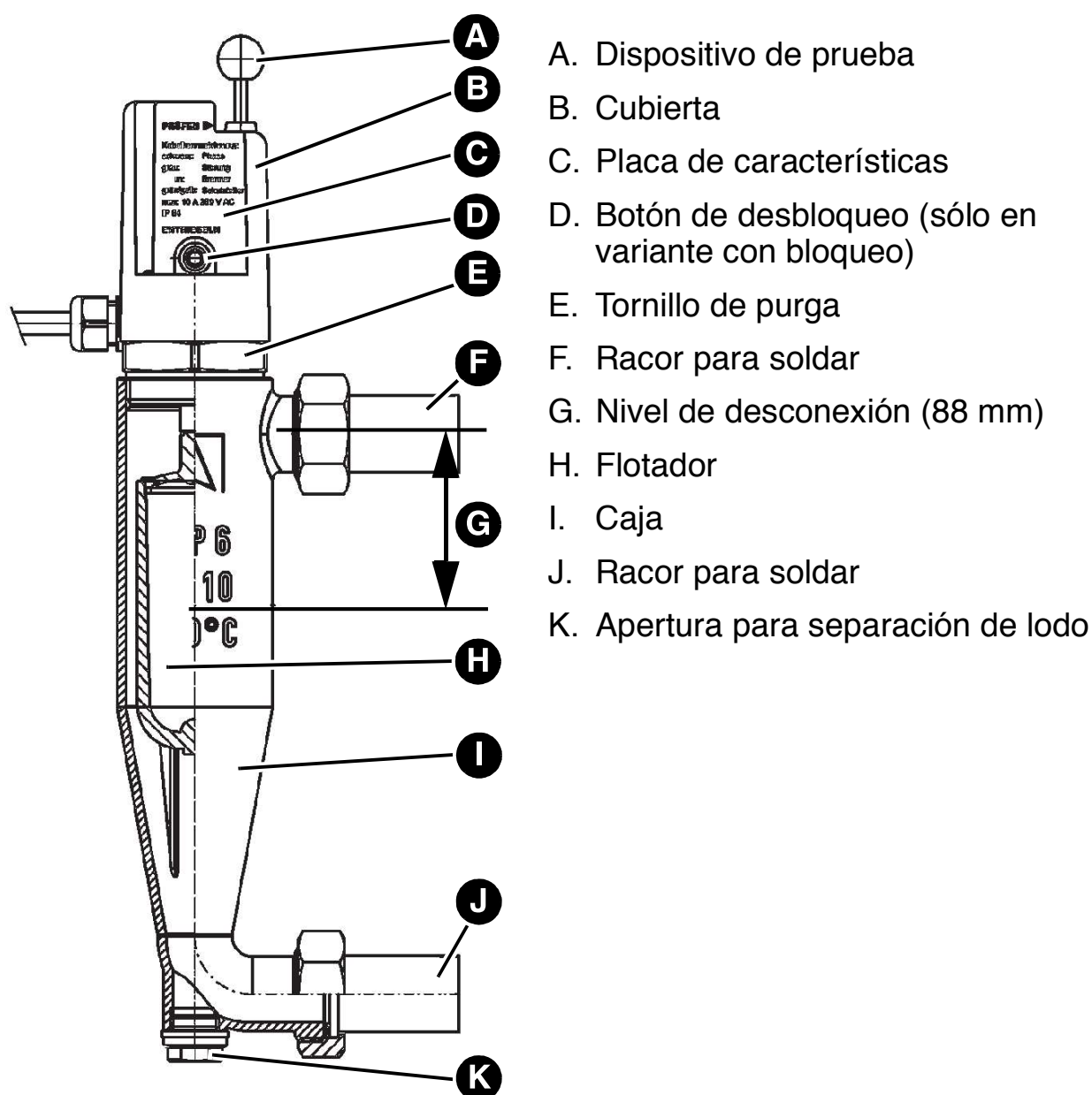
Figura 1: Estructura WMS-WP6
