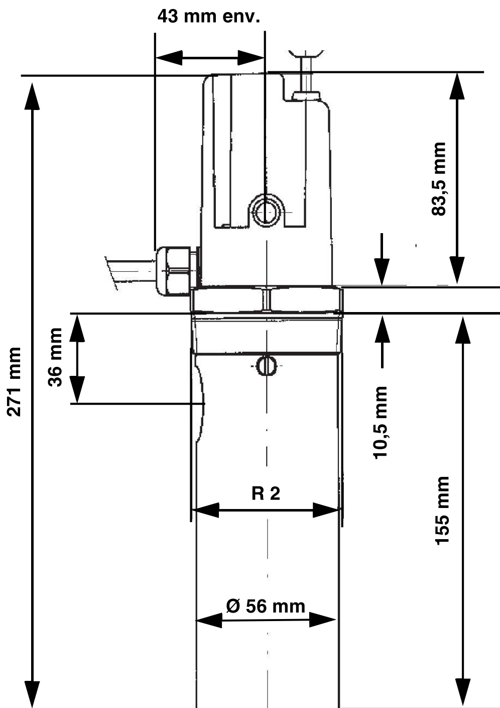
Figure 4: WMS-WP6 avec tube de protection court
