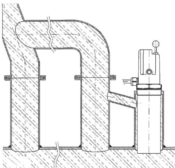
Figura 6: WMS-WP6 con pozzetto corto
