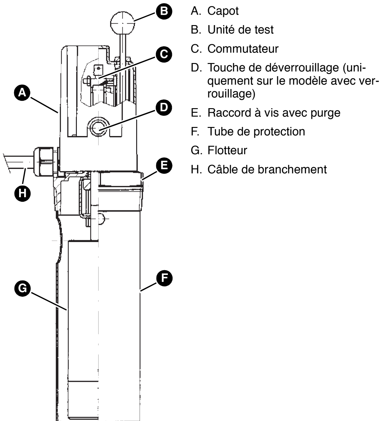
Figure 2: WMS-WP6 avec tube de protection court
