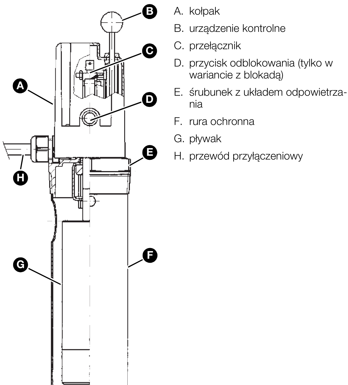
Ilustracja 2: WMS-WP6 z krótką rurą ochronną
