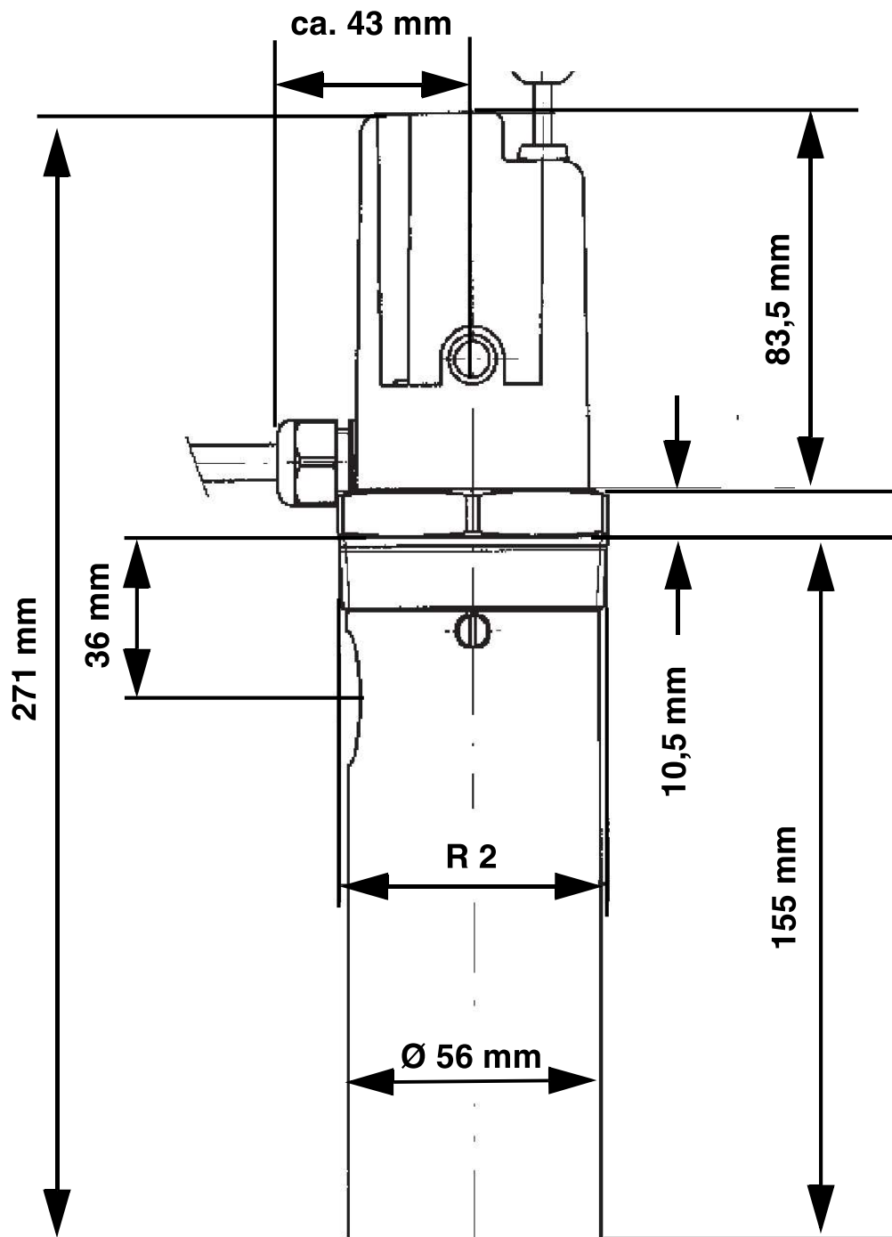
Abbildung 4: WMS-WP6 mit kurzem Schutzrohr
