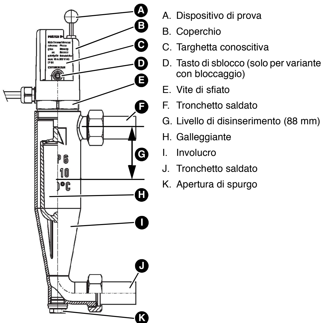
Figura 1: Struttura WMS-WP6
