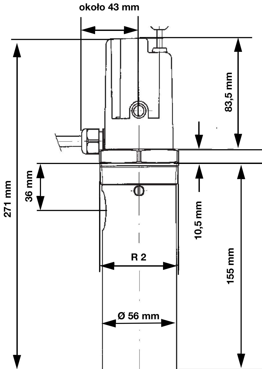
Ilustracja 4: WMS-WP6 z krótką rurą ochronną
