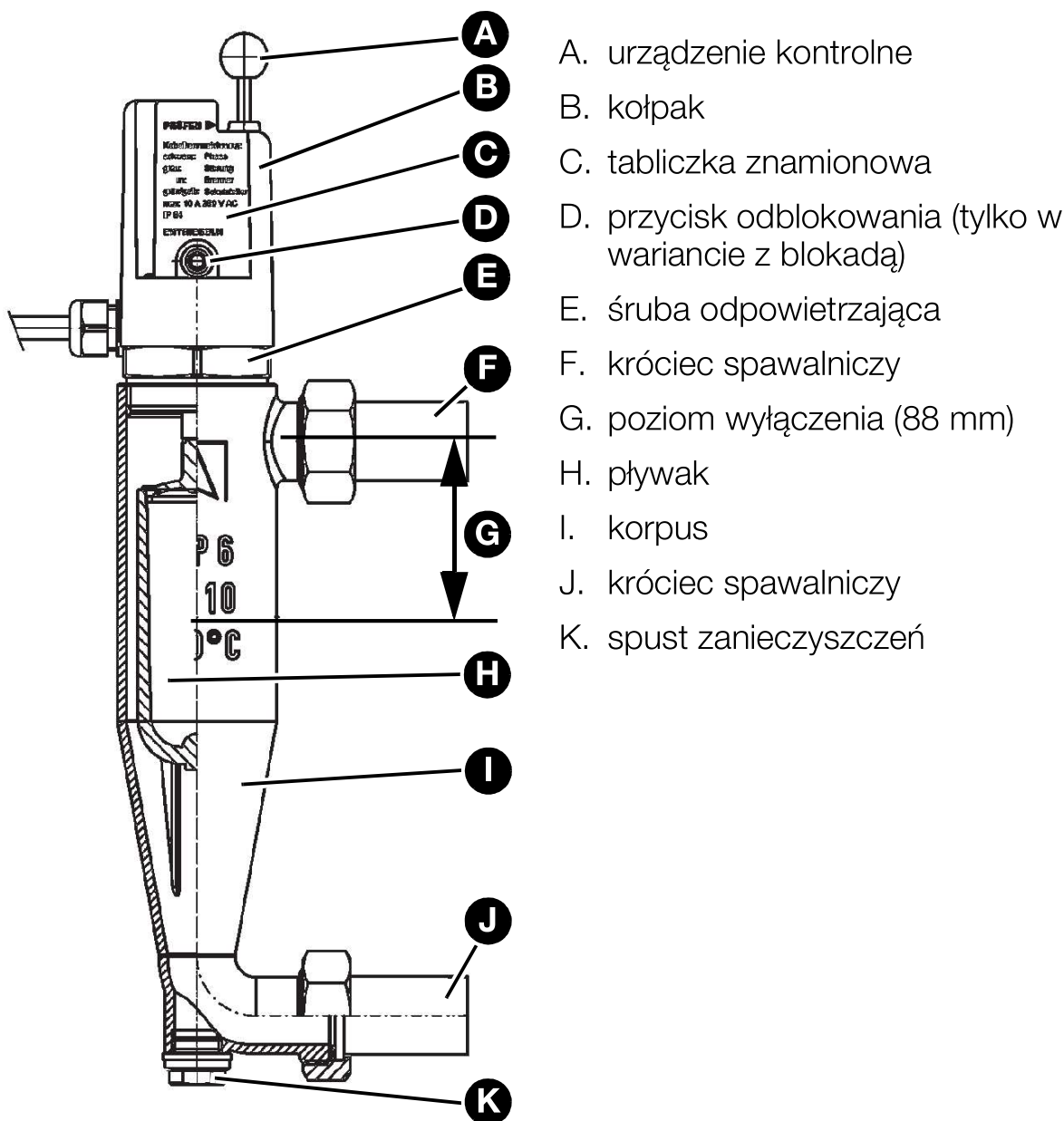
Ilustracja 1: Układ WMS-WP6
