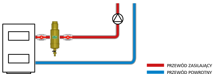
Przykładowa instalacja z obiegiem bezpośrednim
