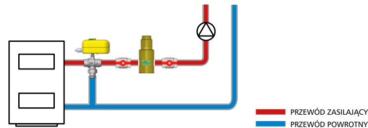
Przykładowa instalacja z zaworem mieszającym
