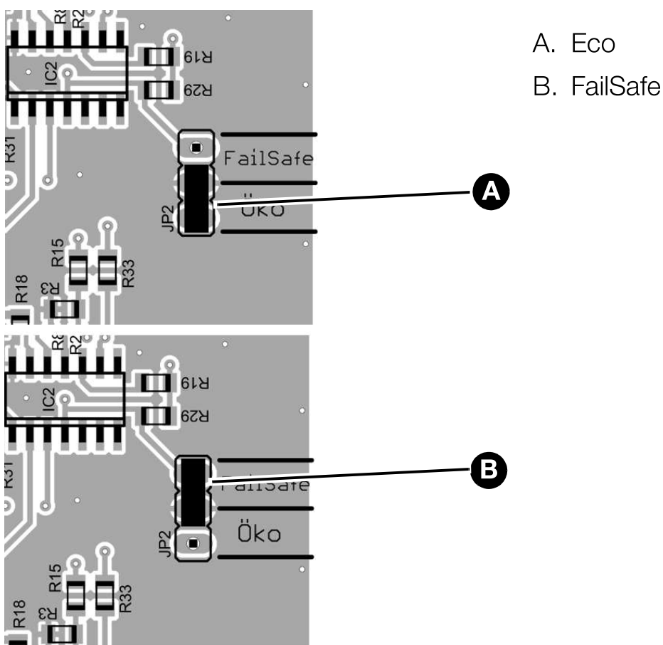
Ilustracja 6: Ustalanie trybu pracy
