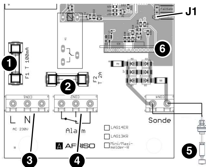
Abbildung 5: Elektrischer Anschluss
