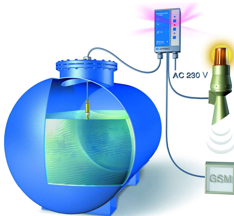
Figure 4: Utilisation standard Maximelder-R
