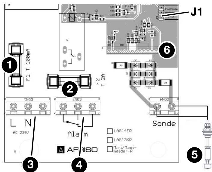
Ilustracja 5: Przyłącze elektryczne
