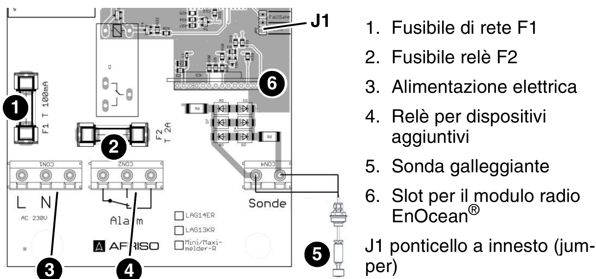
Figura 5: Allacciamento elettrico
