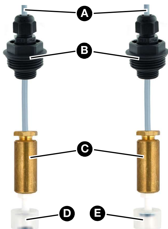
Ilustracja 1: Sonda pływakowa
