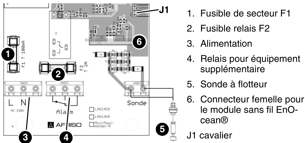
Figure 5: Branchement électrique
