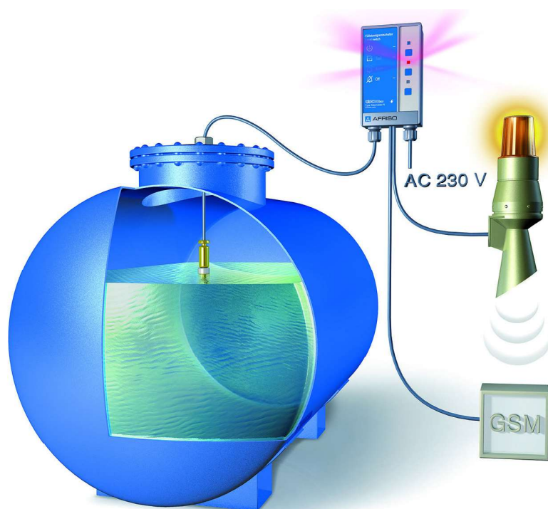
Ilustracja 4: Zastosowanie standardowe Maximelder-R
