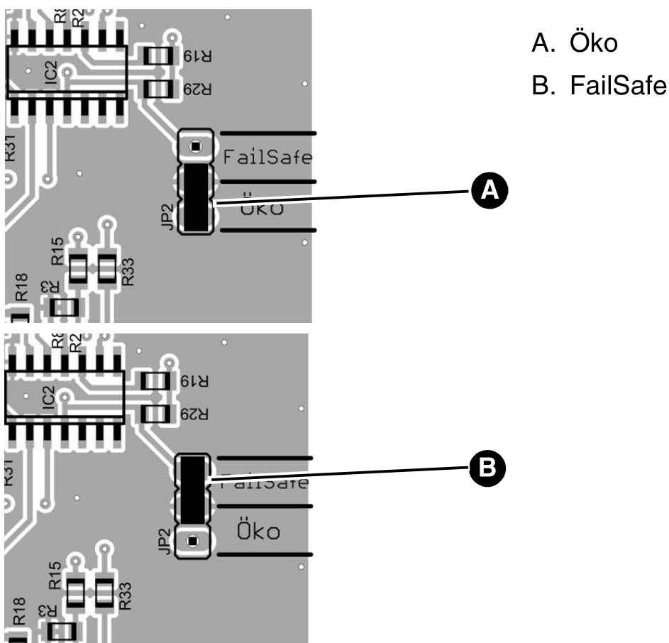
Figura 6: Determinare la modalità di esercizio
