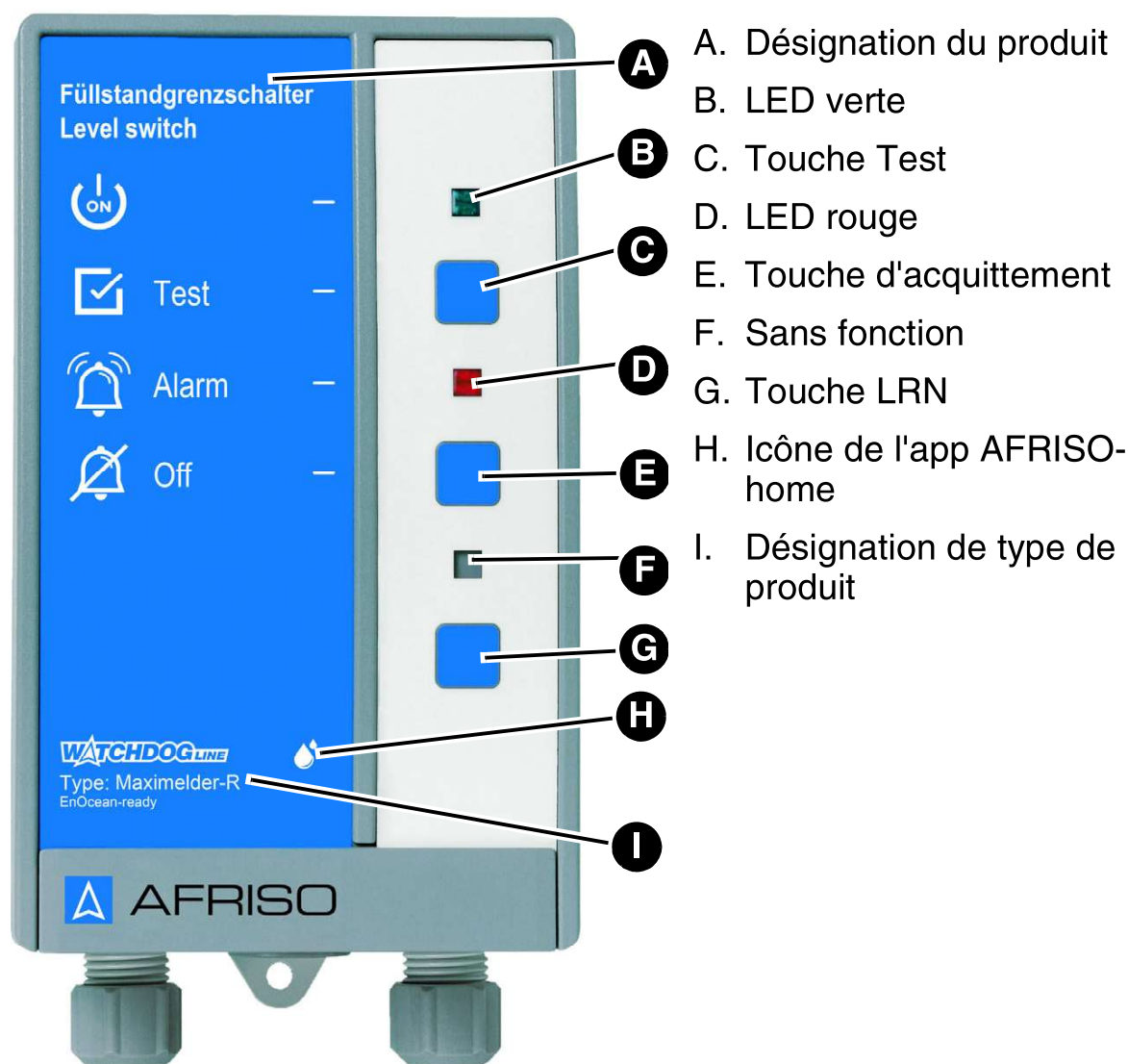
Figure 2: Unité de commande
