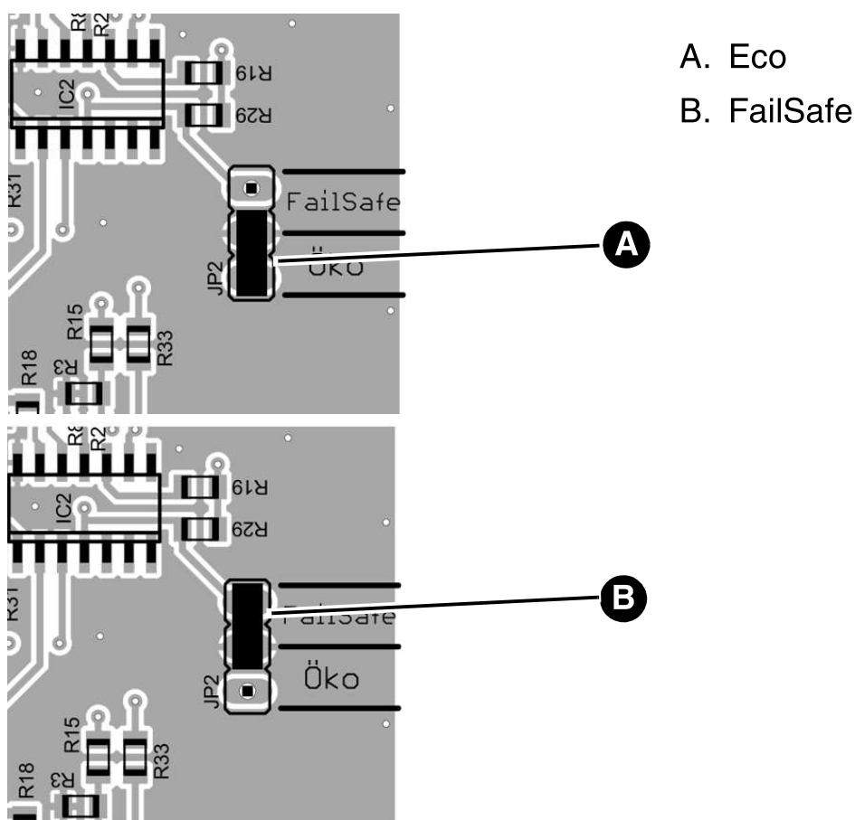
Figure 6: Régler le mode de fonctionnement
