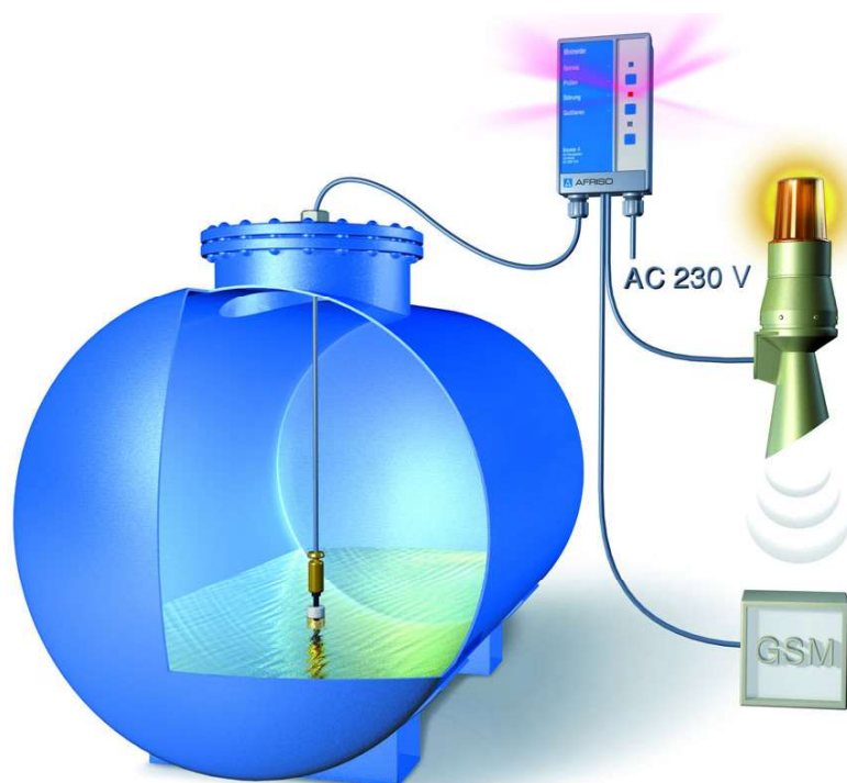
Ilustracja 3: Zastosowanie standardowe Minimelder-R
