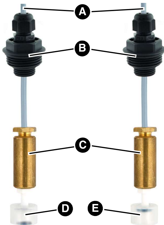
Abbildung 1: Schwimmersonde
