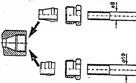
Rys. 7. Schemat montażu rury ssącej z wykorzystaniem zestawu złączek zaciskowych.
