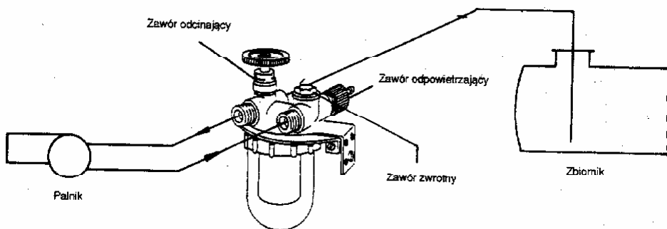
Rys. 6. Schemat podłączenia filtra do instalacji jednorurowej z doprowadzeniem strumienia powrotnego.
