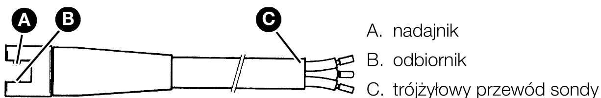
Ilustracja 1: sonda optoelektroniczna
