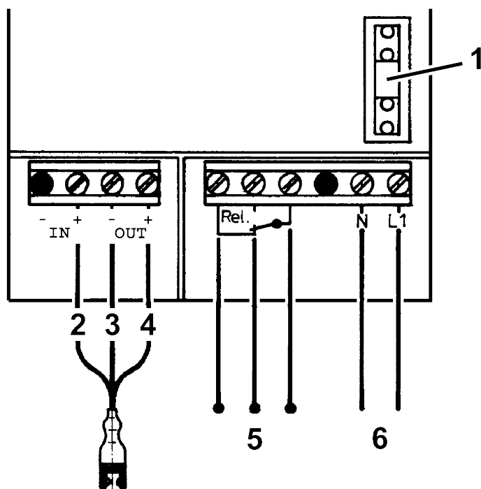
Figura 8: Allacciamento elettrico OM 1
