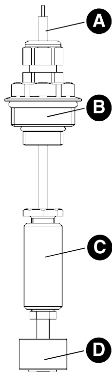
Figura 2: Sonda galleggiante (solo per OM 5+1)
