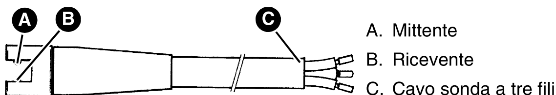
Figura 1: Sonda fotoelettrica
