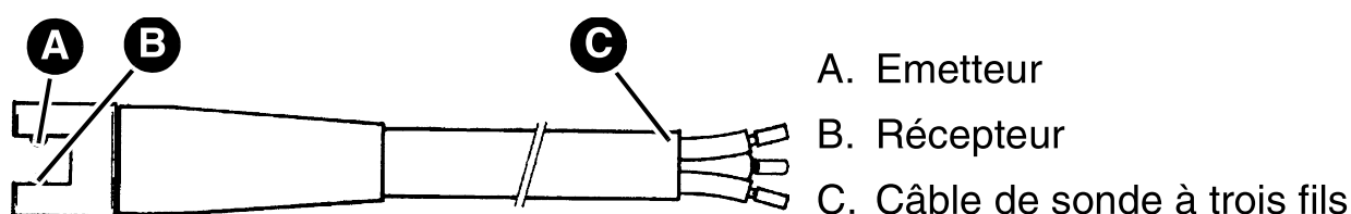
Figure 1: Sonde optoélectronique
