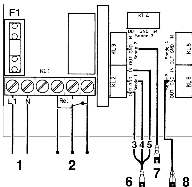
Figura 6: Allacciamento elettrico OM 5
