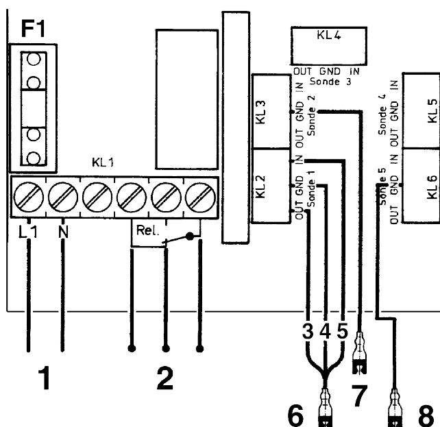
Ilustracja 6: Przyłącze elektryczne OM 5
